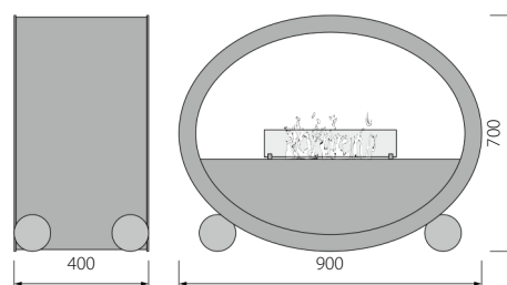
Krea Opal als Standgerät mit Füßen
