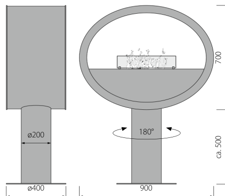
Krea Opal als Standgerät mit Standfuss
